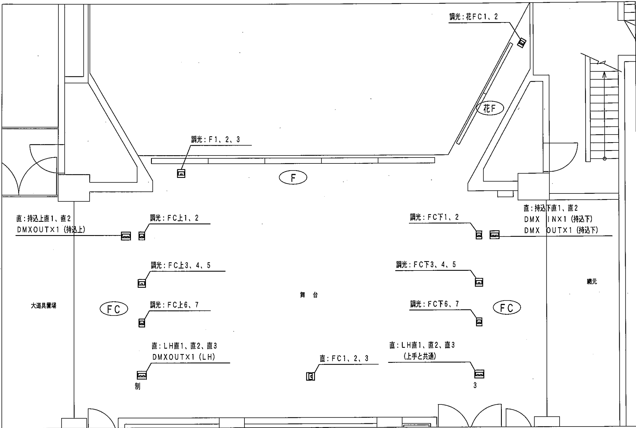
甲山会館 フロアコンセント回路図
